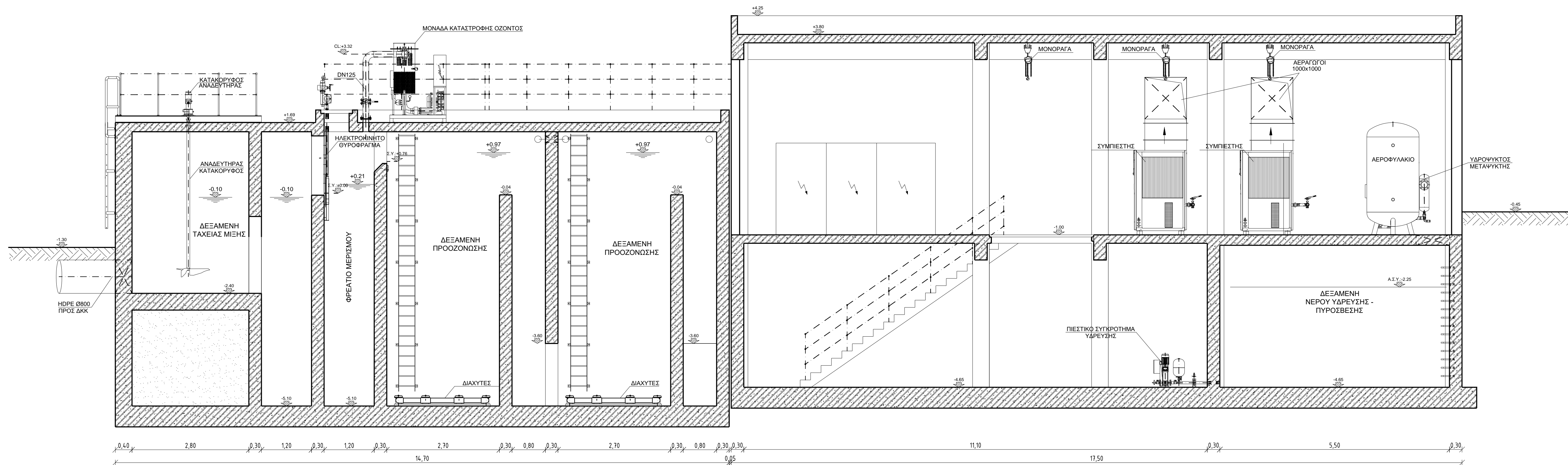
ΤΟΜΗ Α-Α ΚΛΙΜΑΚΑ 1:50
