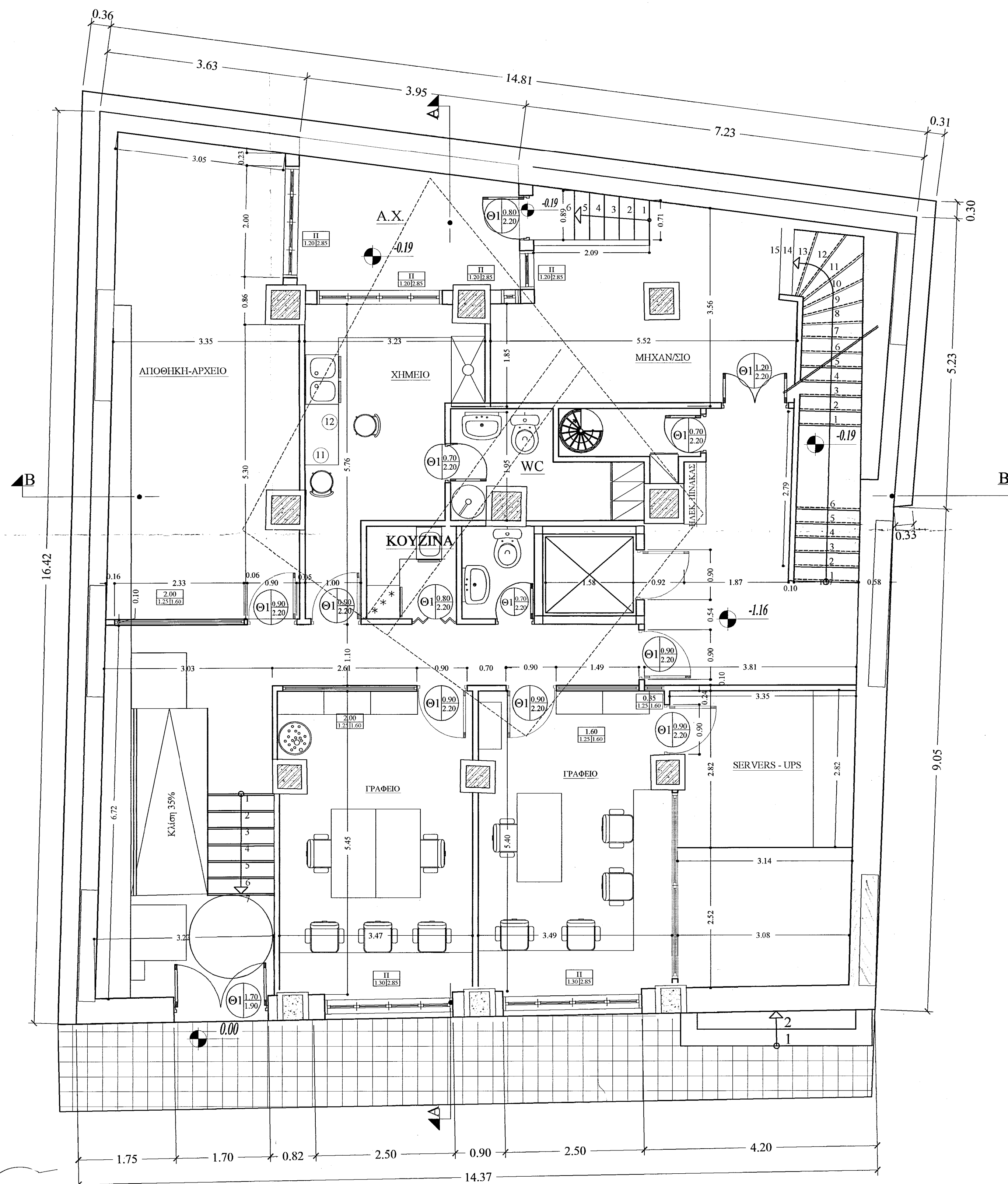
ΚΑΤΟΨΗ ΥΠΟΓΕΙΟΥ ΚΛΙΜΑΚΑ 1/50
