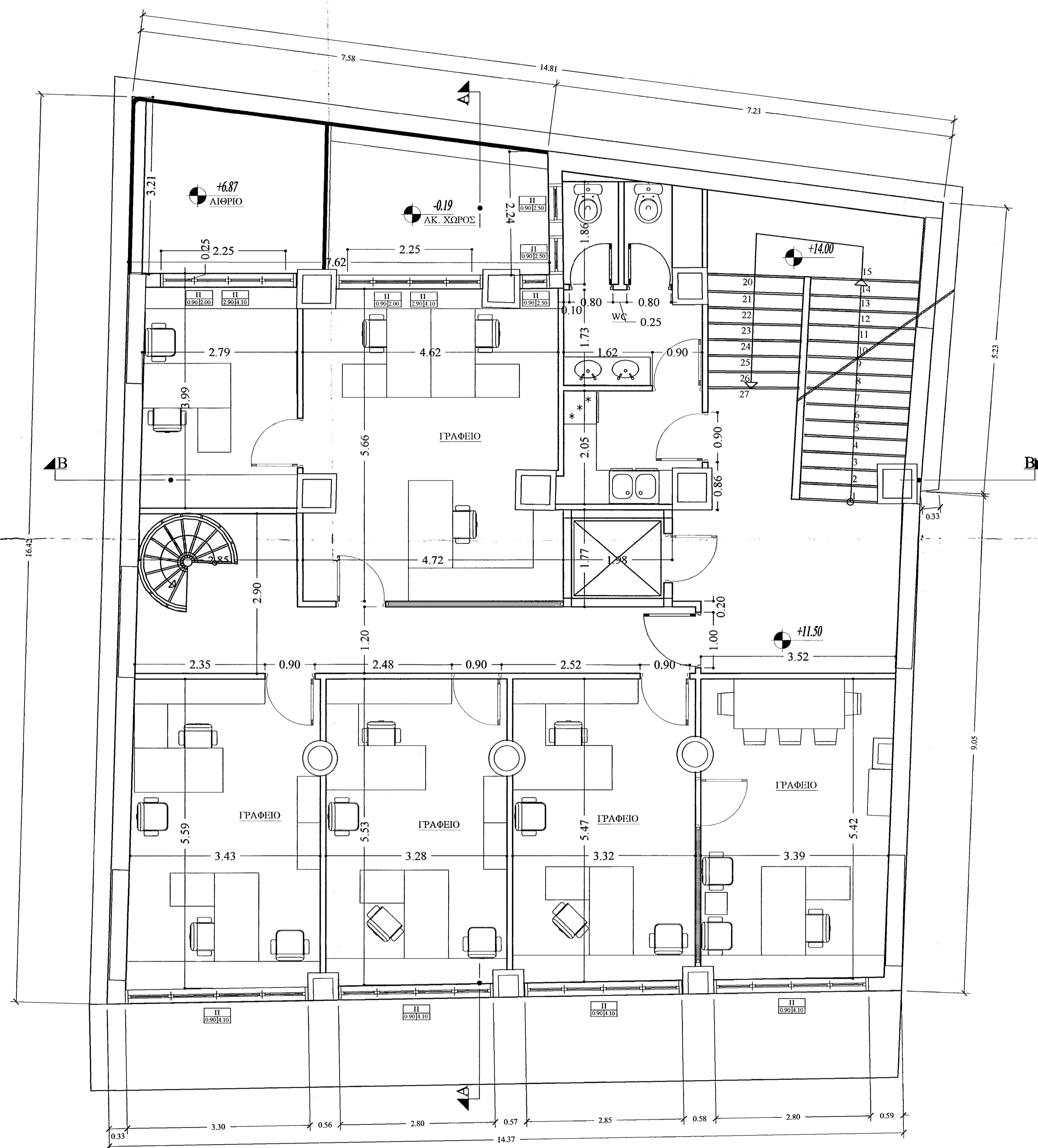
ΚΑΤΟΨΗ Β' ΟΡΟΦΟΥ ΚΛΙΜΑΚΑ 1/50
