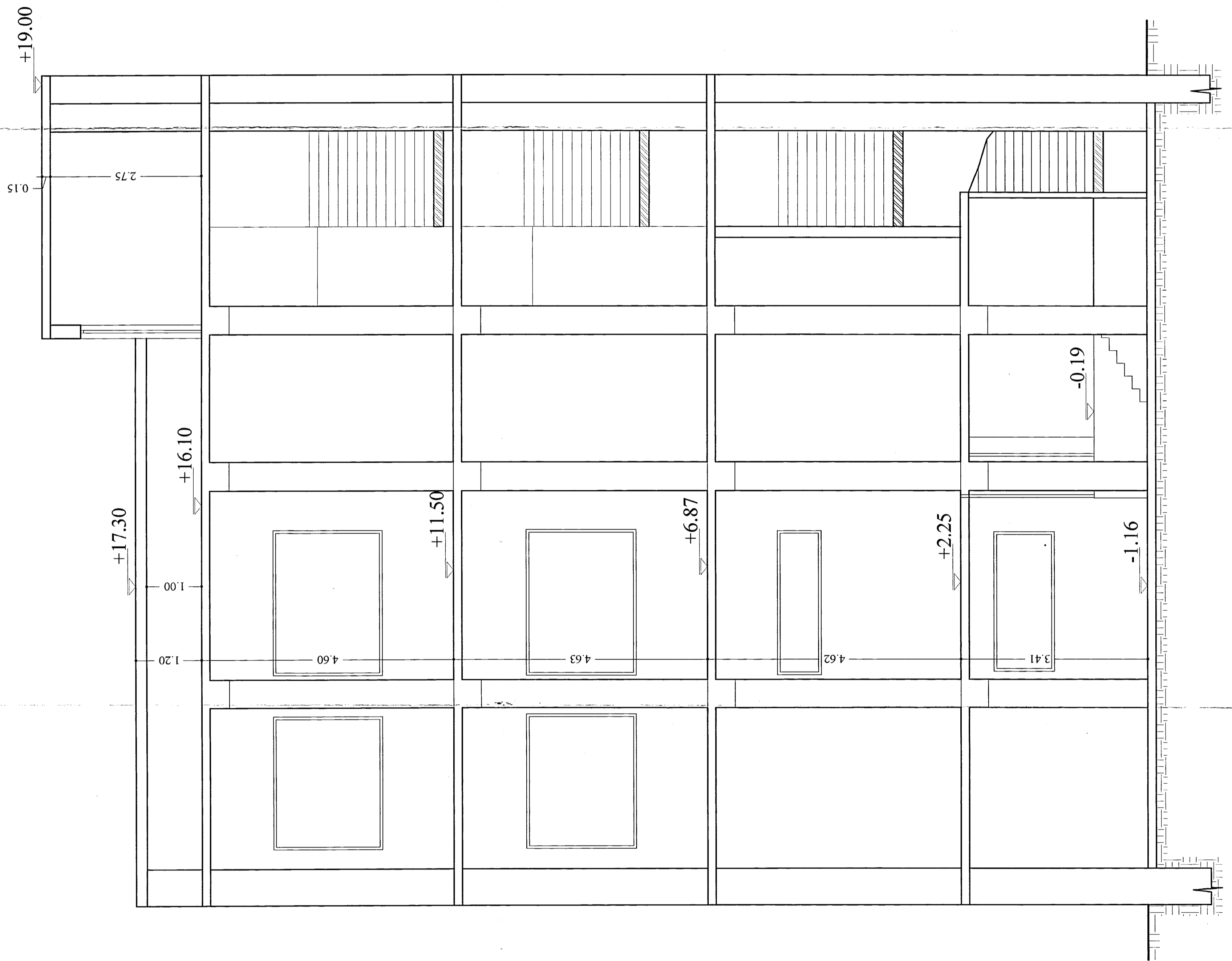
ΤΟΜΗ Β-Β ΚΑΙΜΑΚΑ 1/50
