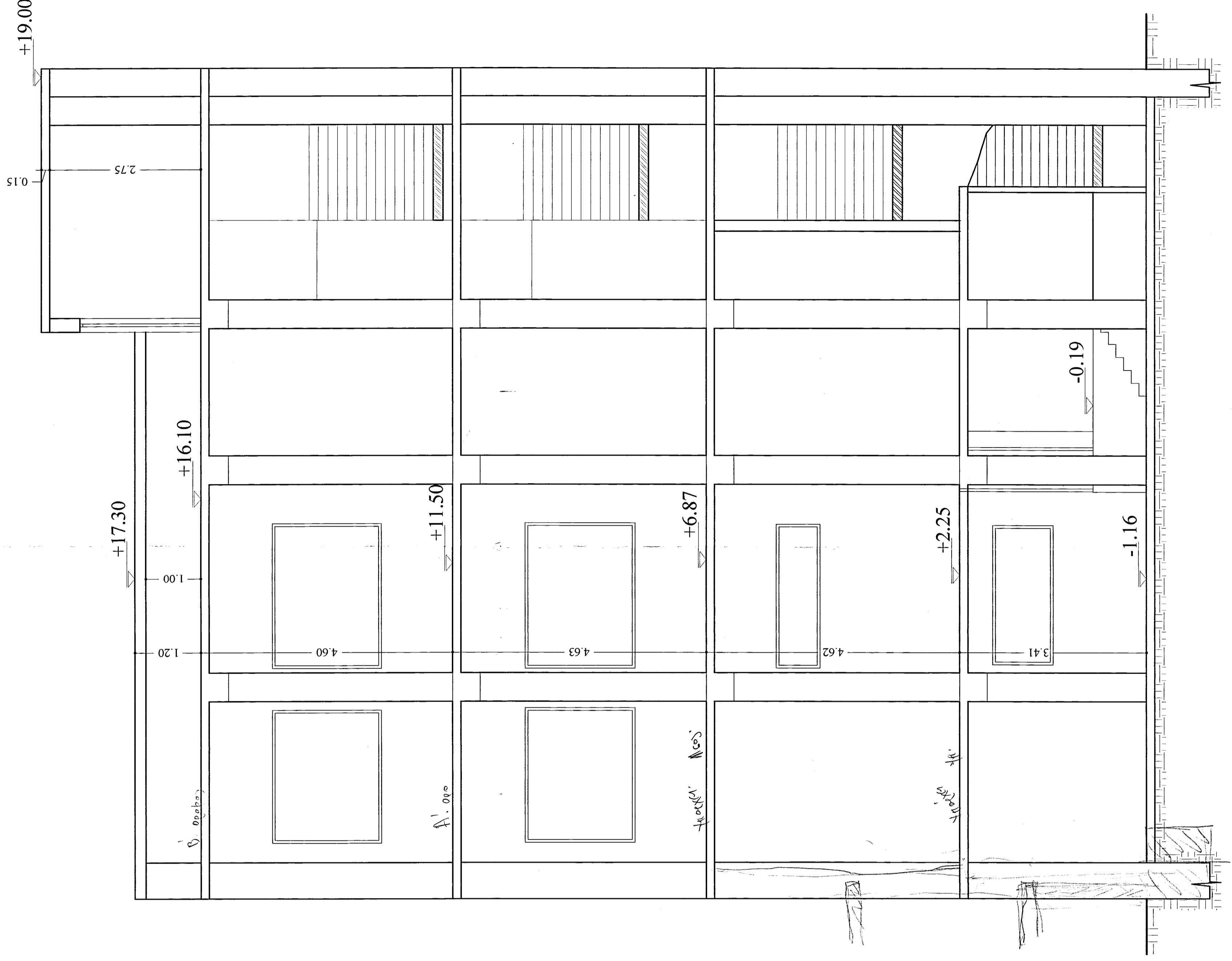
ΤΟΜΗ Γ-Γ ΚΑΙΜΑΚΑ 1/50
